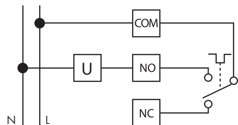
Esquema eléctrico
