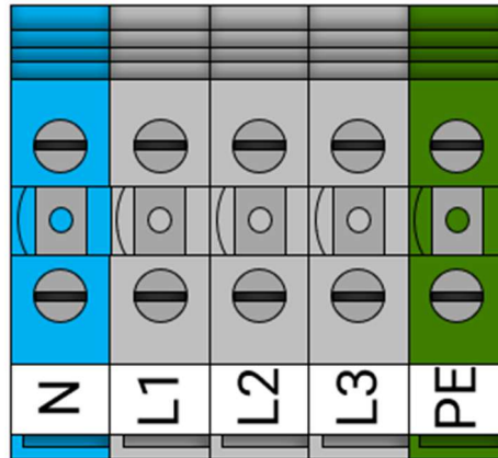
Conexión trifásica
