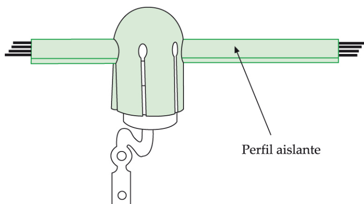
Capuchón aislante para recubrir conductores en aisladores
