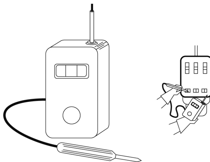
Figura 10. Discriminador de tensión para baja tensión
