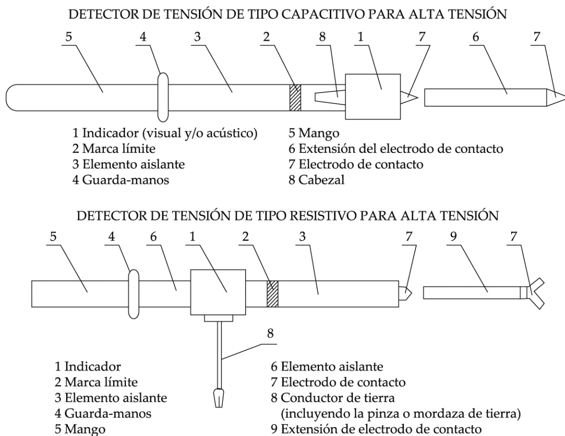
Figura 9. Detectores de tensión para alta tensión
