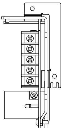
FUENTE DE ALIMENTACIÓN S82J_2524_21A
