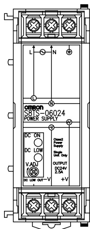
FUENTE DE ALIMENTACIÓN S8TS-06024
