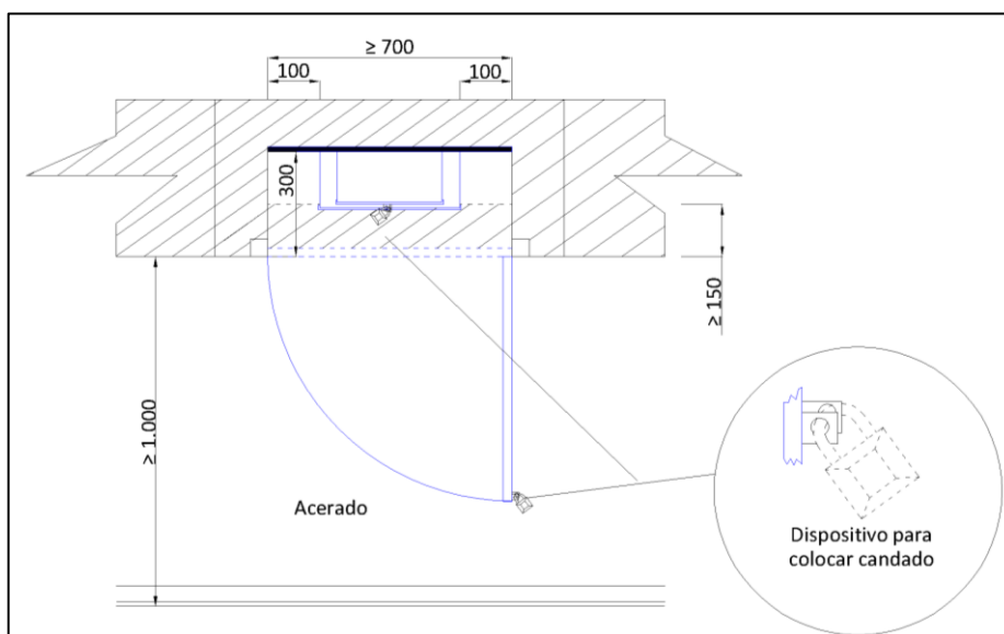
Figura 4. Instalación CGP y CS montaje vertical. Planta.
