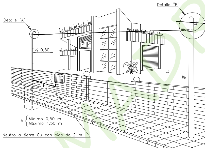
DETALLE "A"
