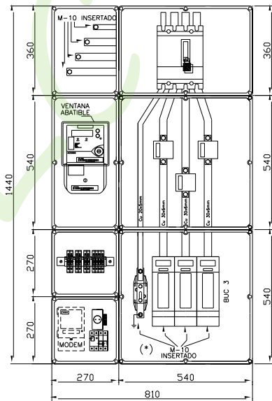
TMF-10 200...400 A
