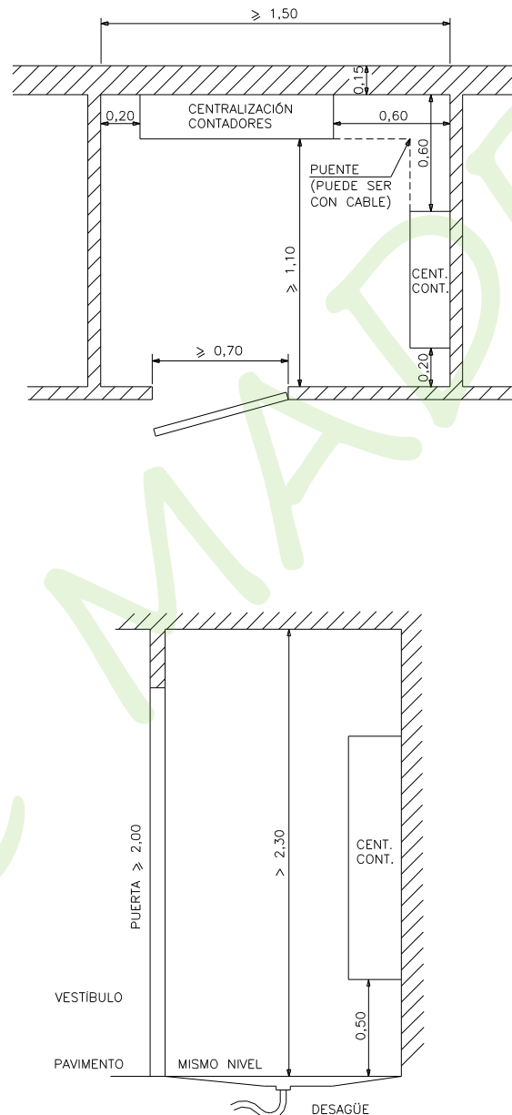
Figura 10. Centralizaciones superiores a 16 contadores en varias paredes
