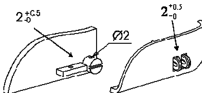
Fig. 6.- Ejemplos de dispositivos para el sistema de precintado
