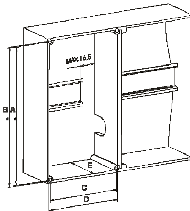
Fig 2.- Caja CCE-ICP 32 y CCS-ICP 40
