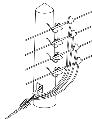
DETALLE "B"
