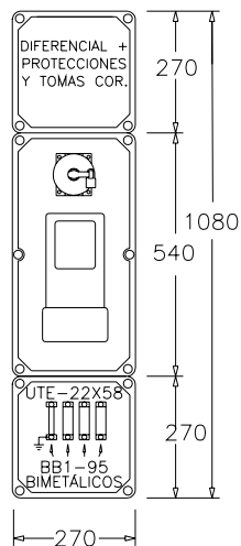
CPMST-T (Trifásico)
