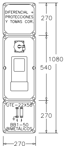
CPMST-M (Monofásico)
