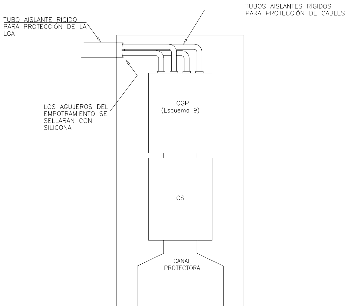
Figura 10. Detalle de la conexión de la línea general de alimentación (LGA) en la CGP
