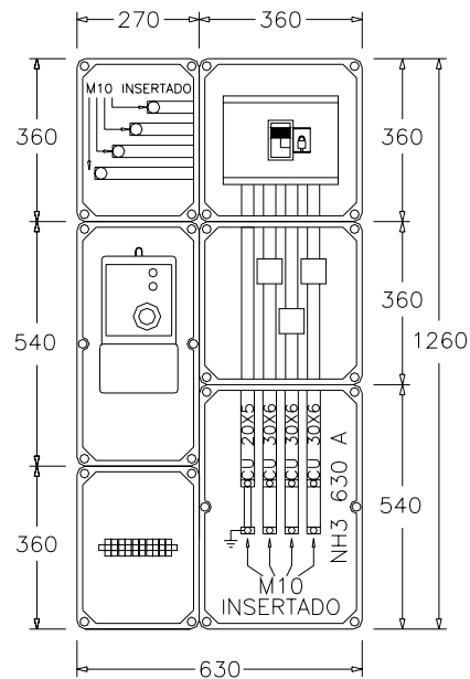
TMF10 200-315 A
