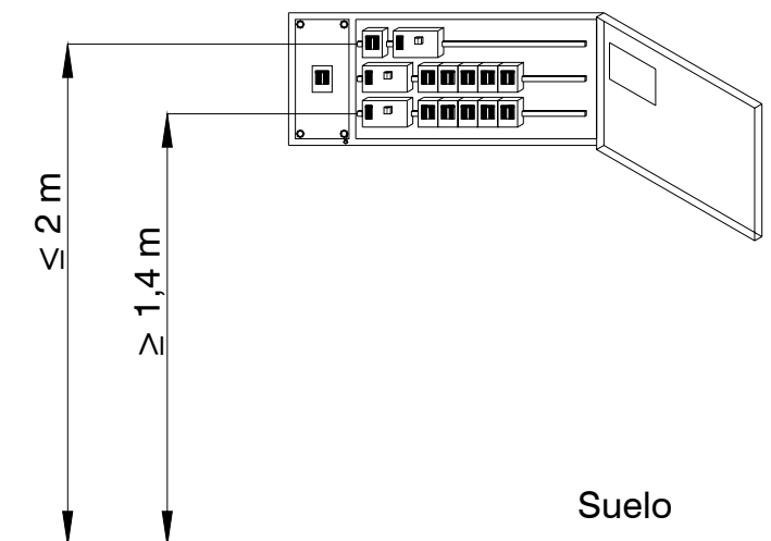
Figura 16. Ubicación del Cuadro General de Mando y Protección
