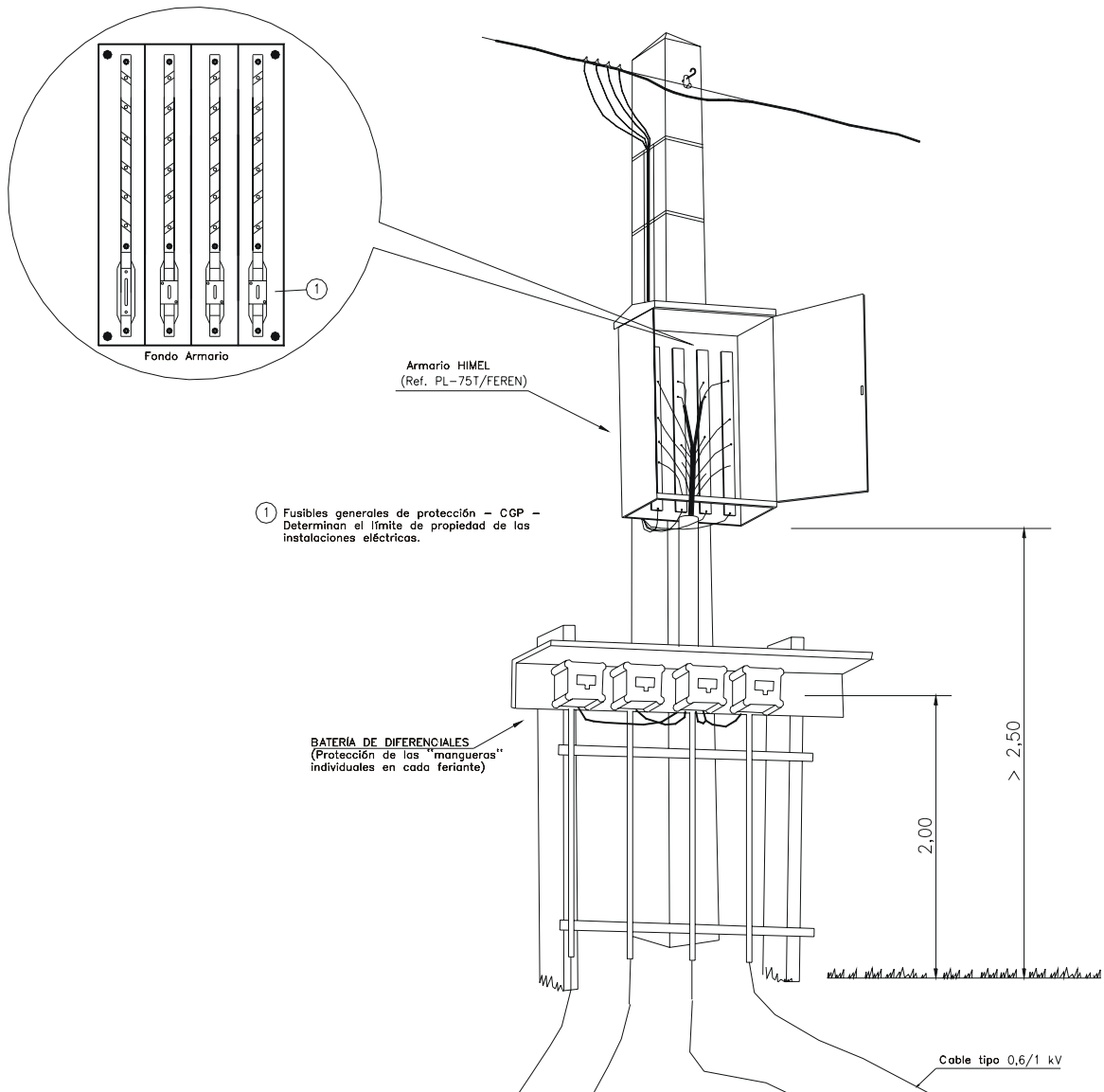
Figura 17. Esquema de suministro a feriantes
