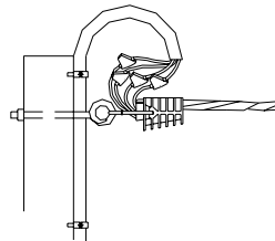
DETALLE "A"
