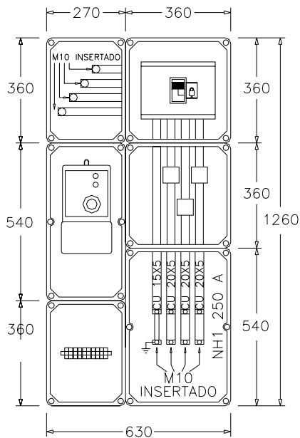
TMF10 80-160 A
