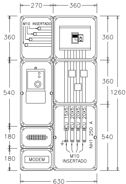
TMF10
