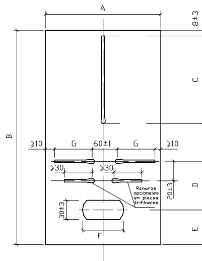
Figura 9. Dimensiones de las placas de montaje de contadores en centralizaciones tipo panel
