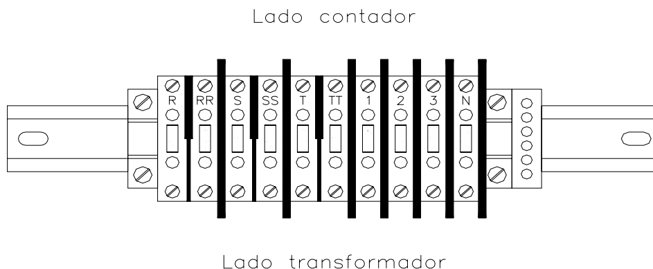
Figura 4. Formación de la regleta
