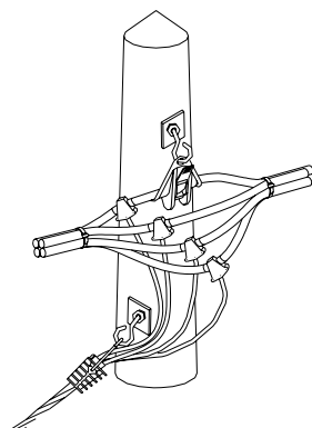
DETALLE "B"
