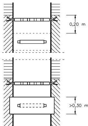
Figura 15. Detalle de instalación de las derivaciones individuales
