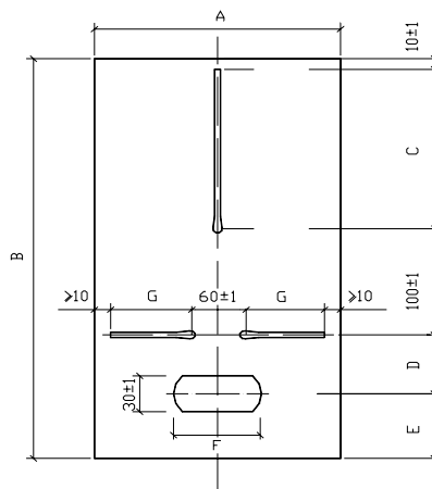
Figura 8. Dimensiones de las placas de montaje de contadores
