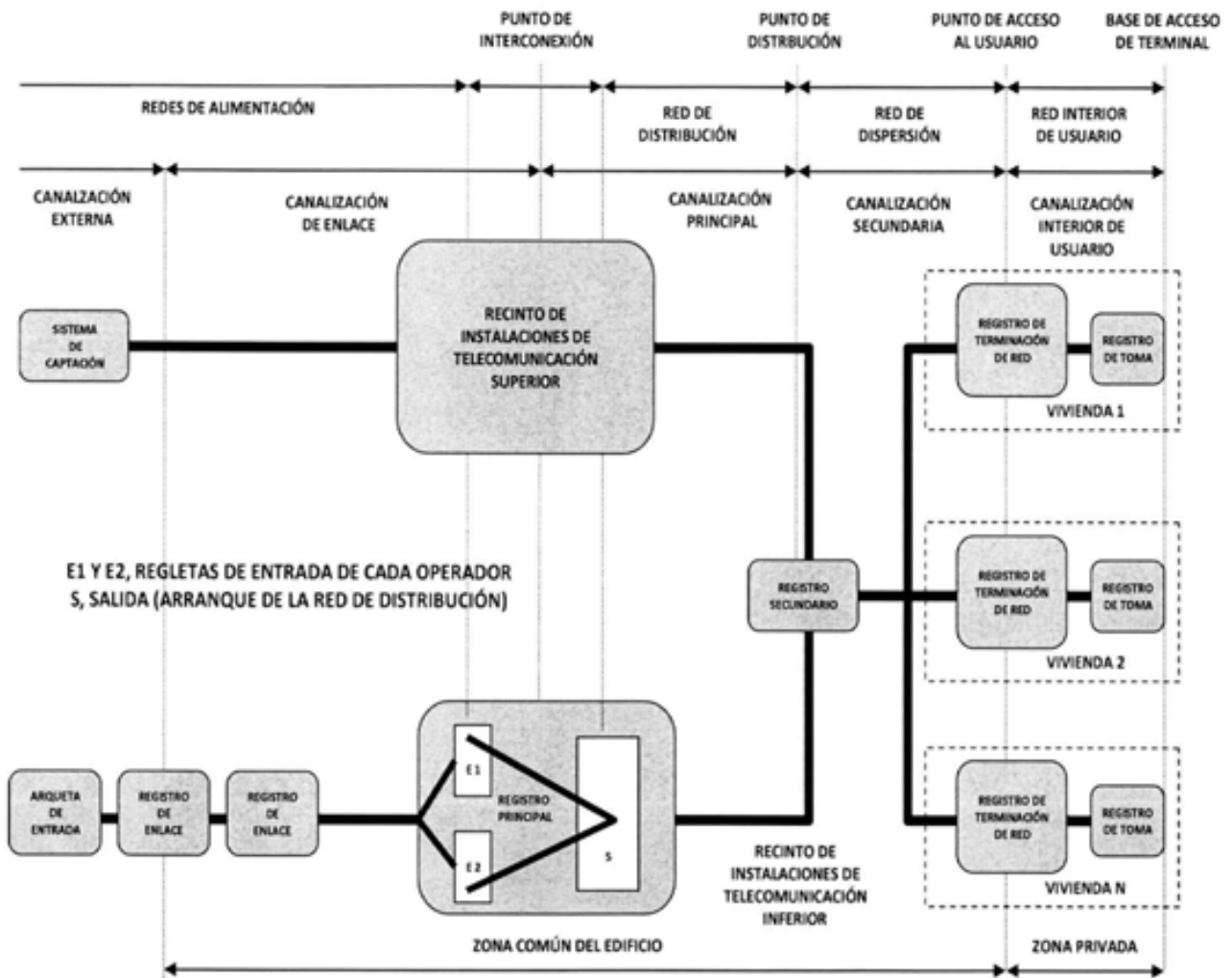
APENDICE 1: Esquema general de una ICT
