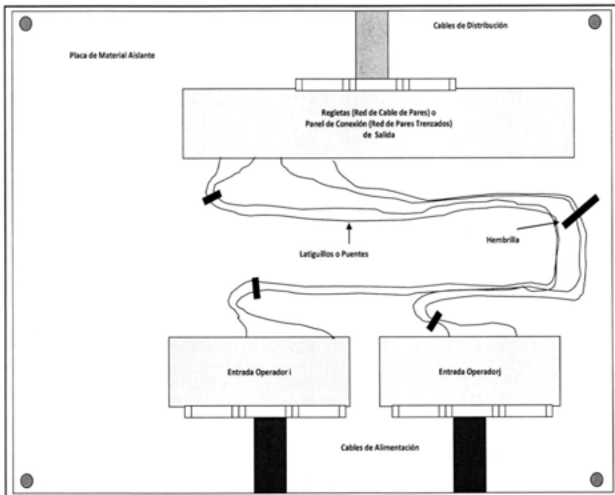
Apéndice 5: Punto de Interconexión de la Red de Pares/Pares Trenzados
