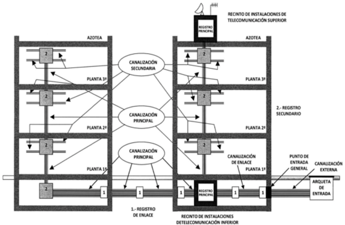
APENDICE 6: Esquema general de canalizaciones con varias verticales en edificios independientes
