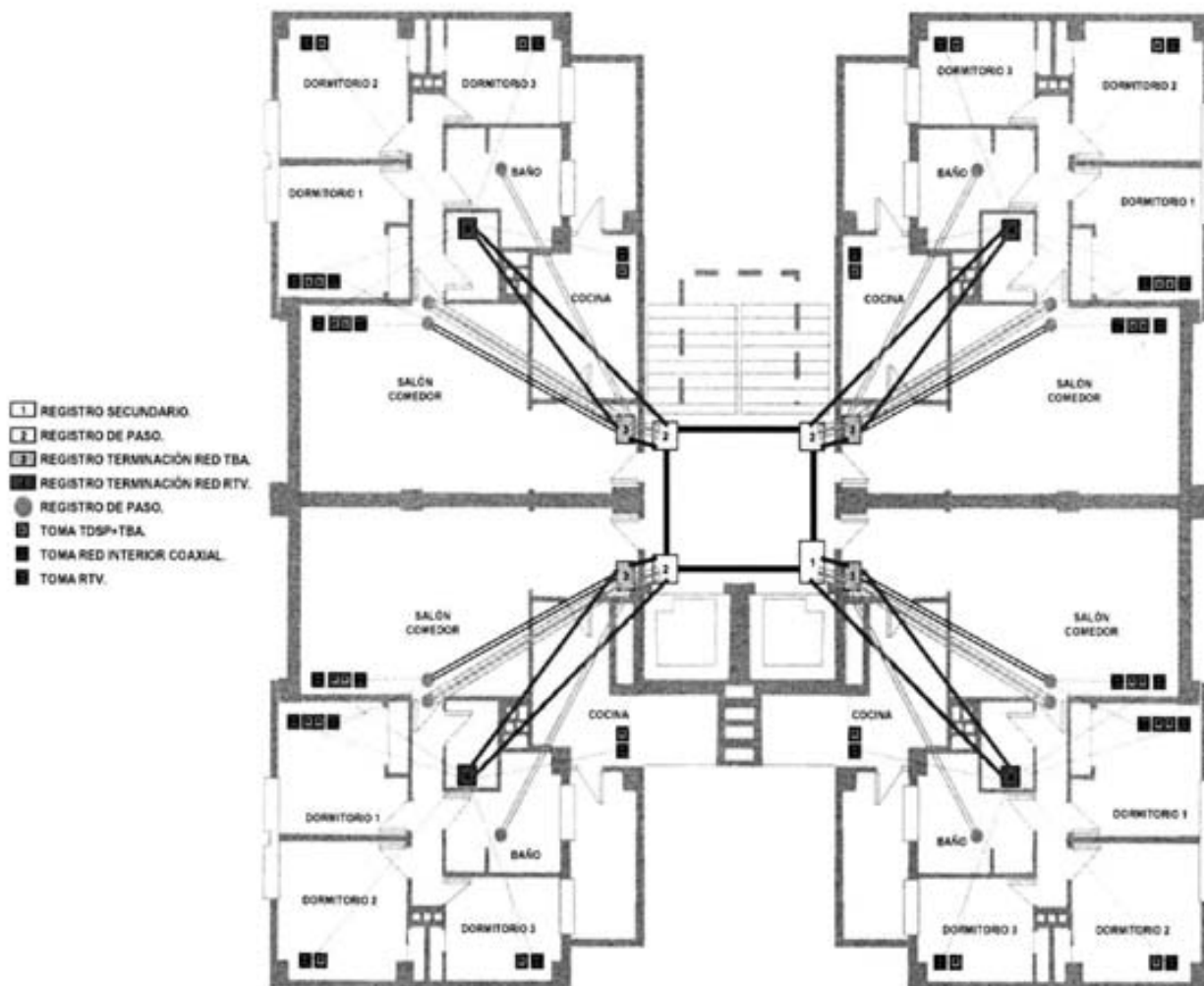
APENDICE 7: Canalización secundaria y red interior de usuario
