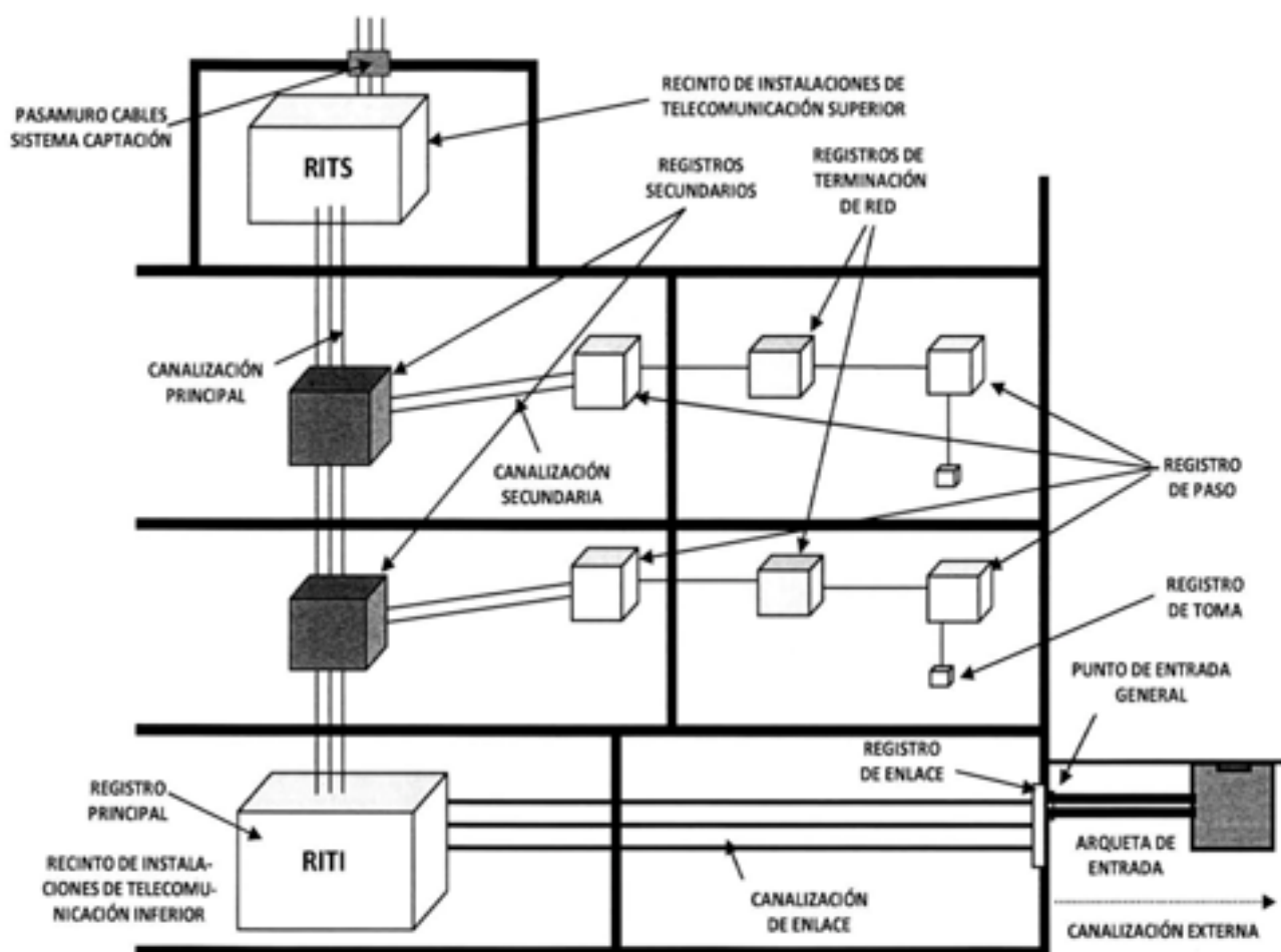
APENDICE 2: Esquema de canalizaciones para inmuebles de pisos
