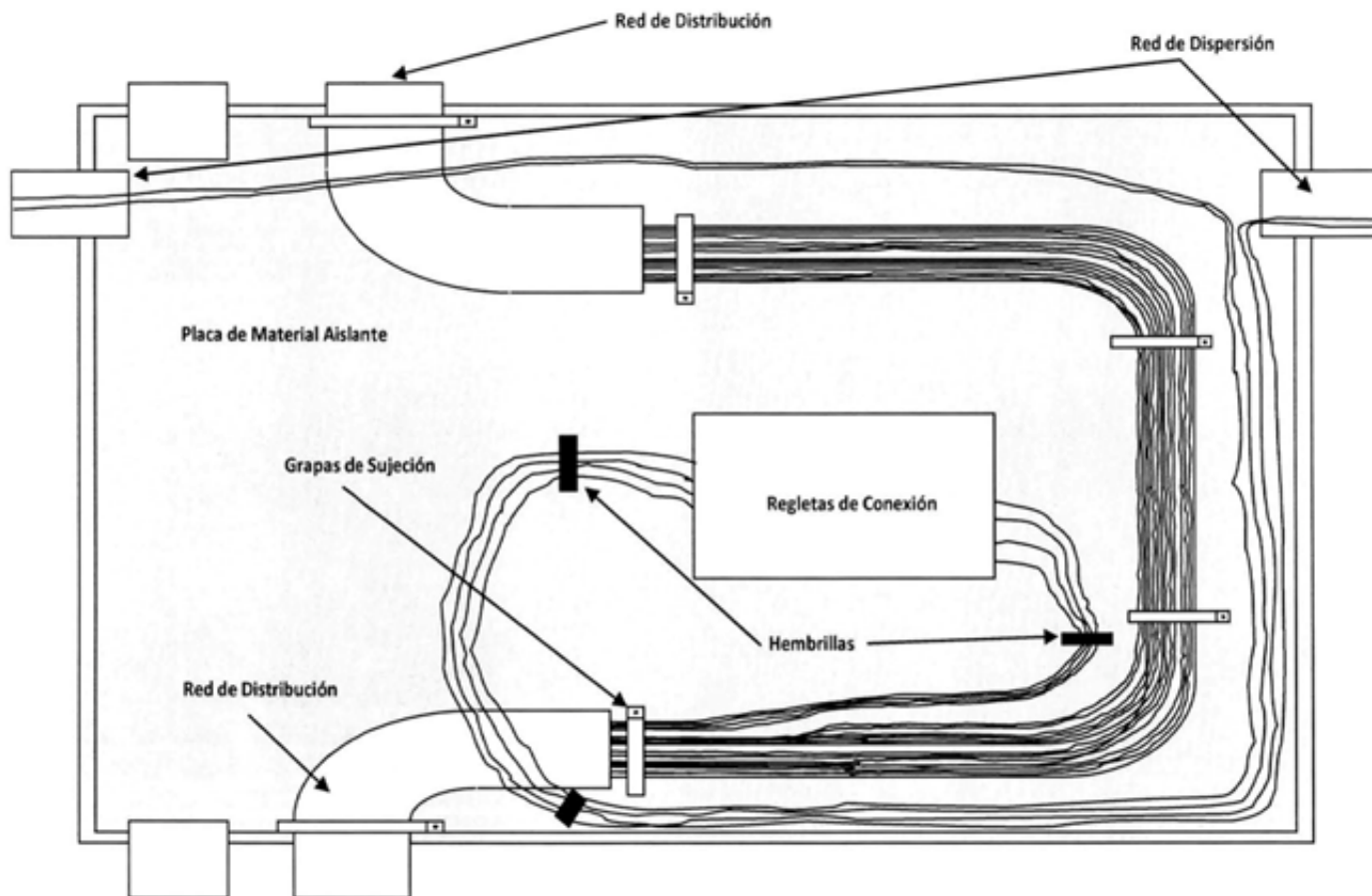
Apéndice 8: Punto de Distribución de la Red de Cable de Pares
