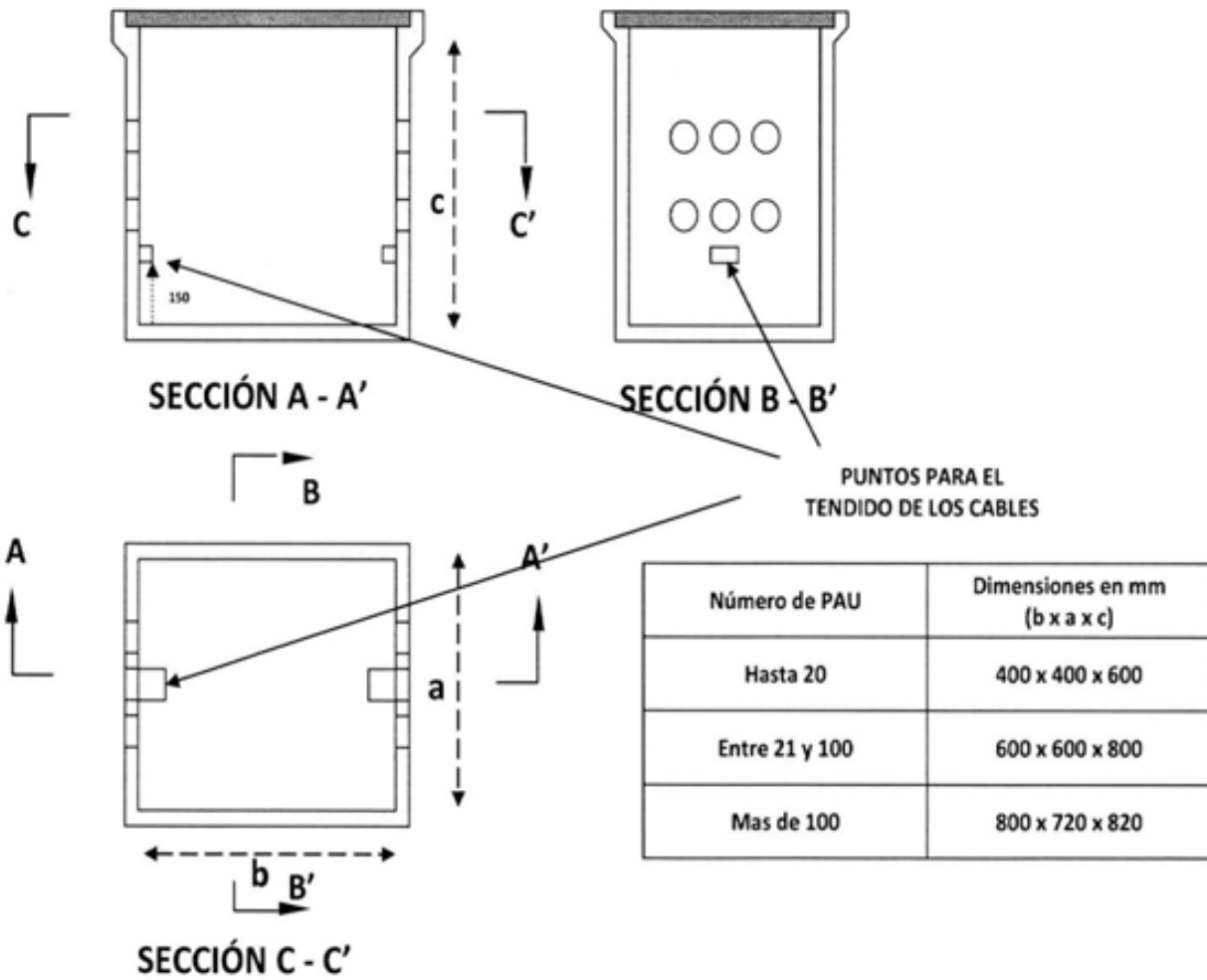
APENDICE 3: Dimensiones mínimas de la arqueta de entrada
