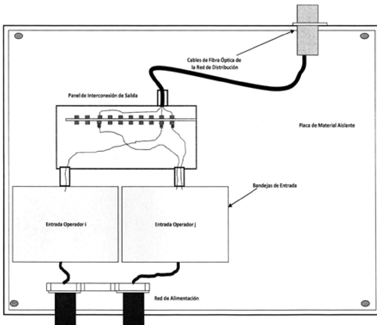
Apéndice 7: Punto de Interconexión de la Red de Cables de Fibra Óptica
