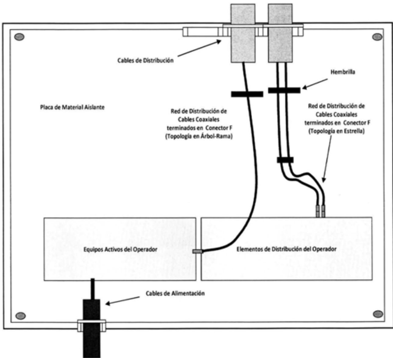
Apéndice 6: Punto de Interconexión de la Red de Cables Coaxiales
