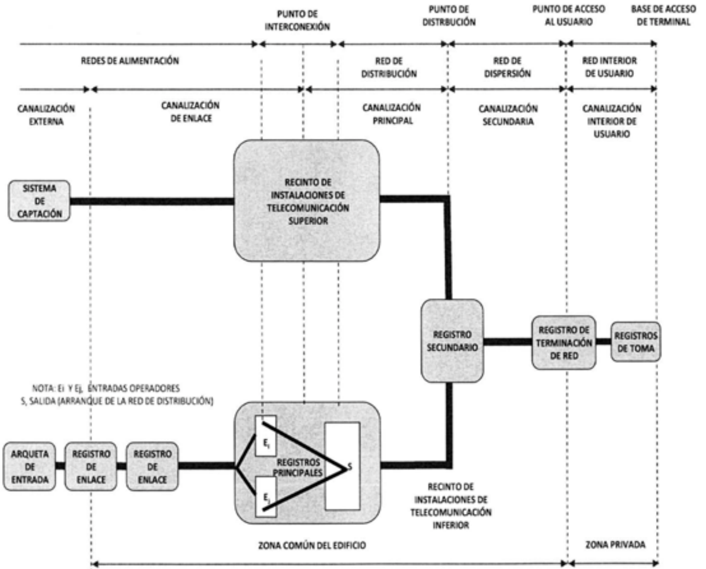
Apéndice 1: Esquema General de una ICT
