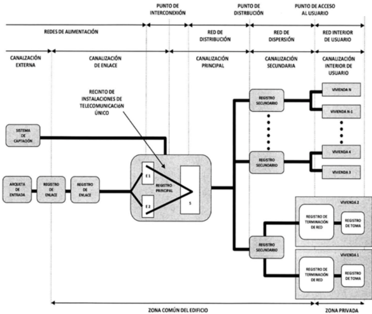
APENDICE 8: Esquema general de la ICT para viviendas unifamiliares
