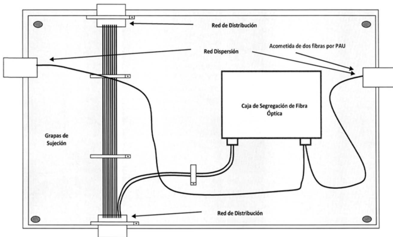
Apéndice 10: Punto de Distribución de Red de Cables de Fibra Óptica
