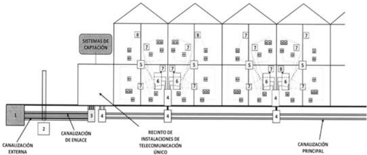
APENDICE 9: Infraestructura para viviendas unifamiliares
