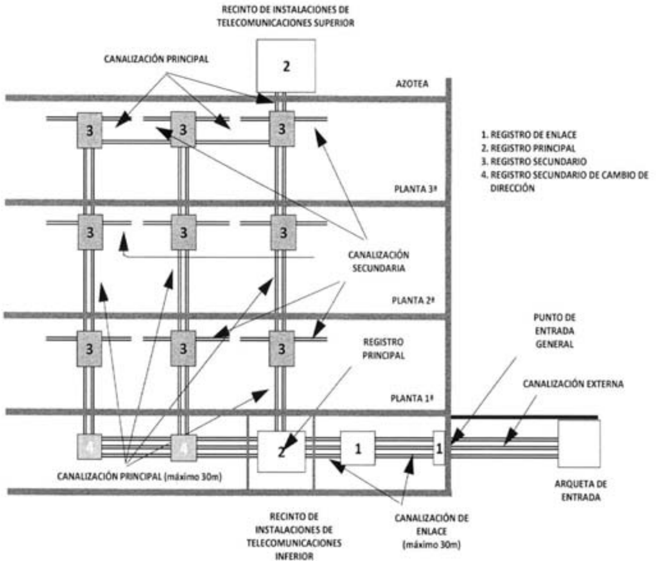
APENDICE 5: Esquema general de canalizaciones con varias verticales
