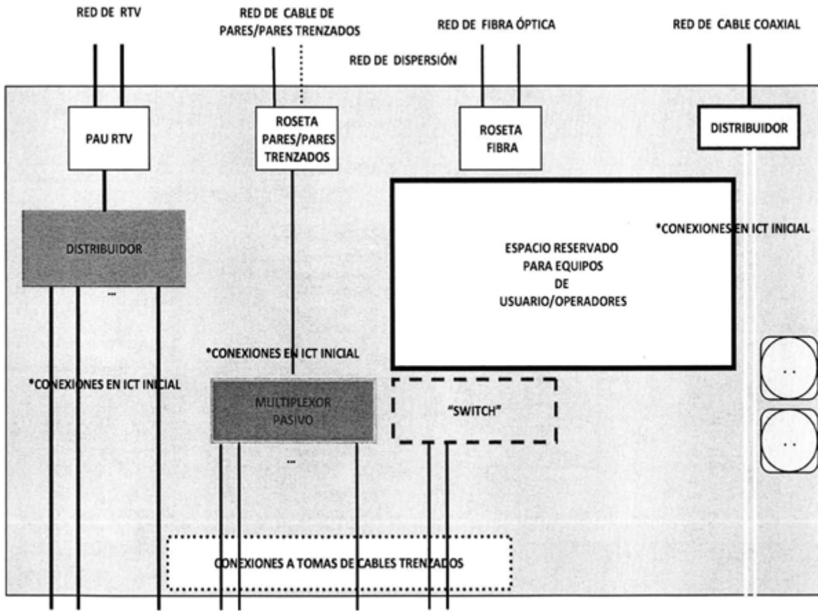
Apéndice 12: Esquema General de Ubicación de Elementos en Registro de Terminación de Red
