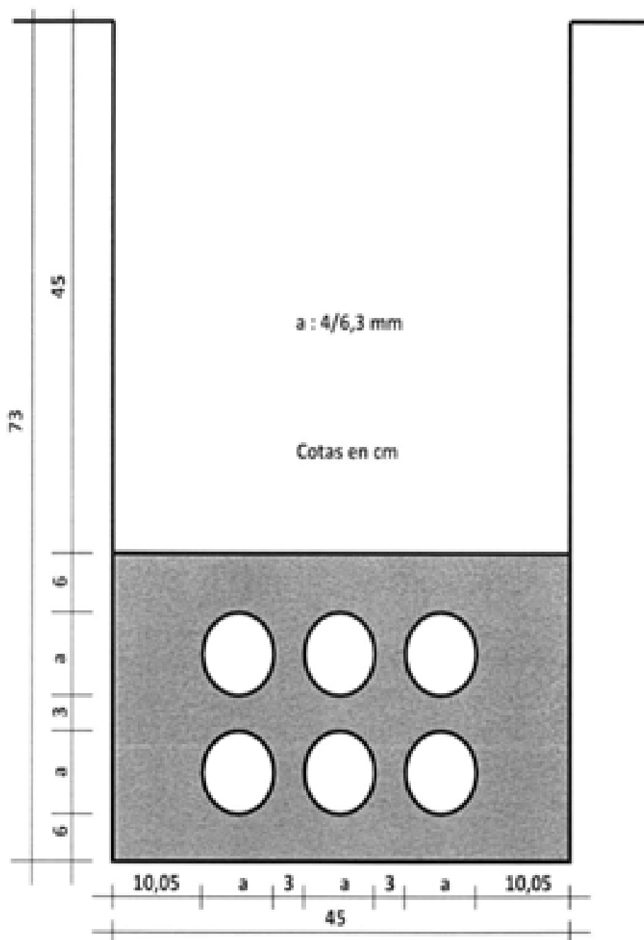
APENDICE 4: Sección transversal de la canalización de enlace
