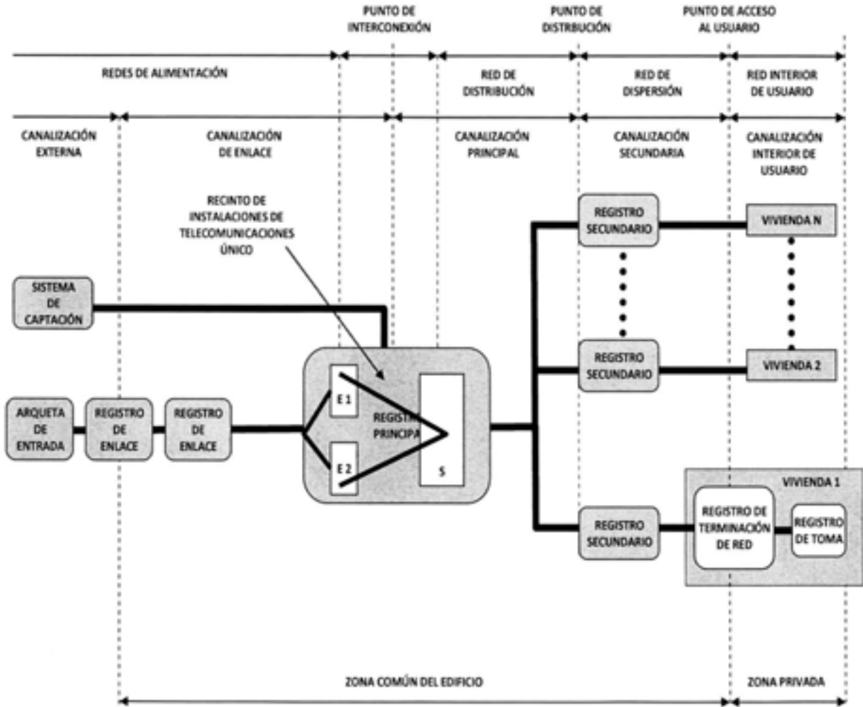
Apéndice 11: Esquema General para agrupaciones de viviendas unifamiliares
