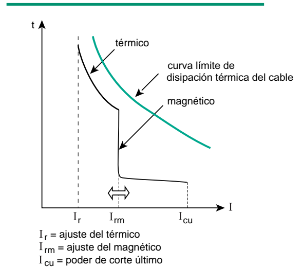
Fig. 5: Curva de disparo de un interruptor automático termomagnético.
