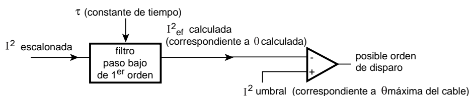
Fig. 7: Realización de la función Largo Retardo LR.
