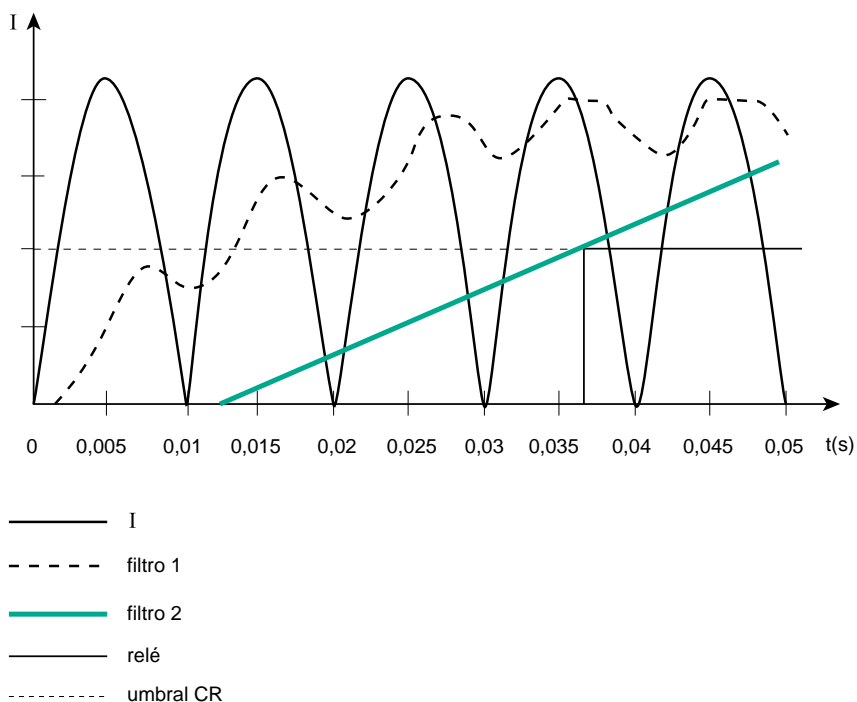
Fig. 16: Defecto persistente.
