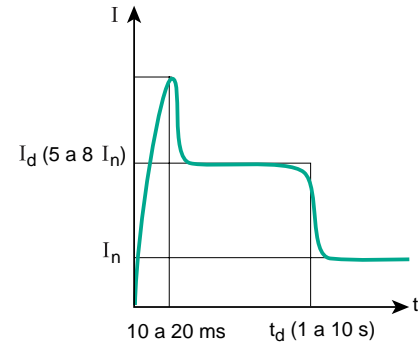
Fig. 14: Conexión de un motor.
