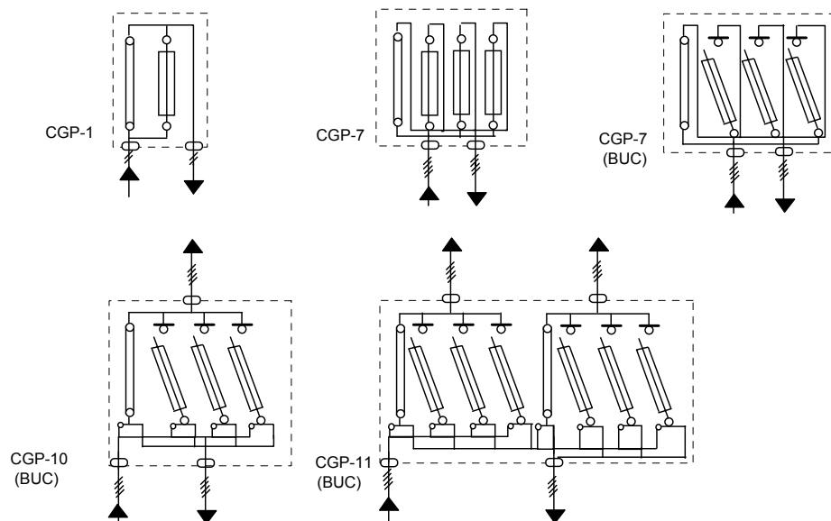
Fig. 1: Esquemas eléctricos de CGP*
