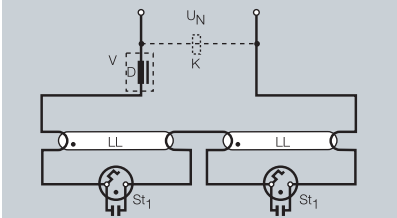
Fig. 2 Conexión en serie para 2 lámparas 4 W, 6 W, 8 W, 15 W, 18 W, 20 W y 22 W a 220. Sólo con cebadores ST 151 + ST 172 (ver página 5.44)
