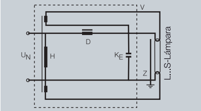
Fig. 4 Encendido rápido inductivo RS
