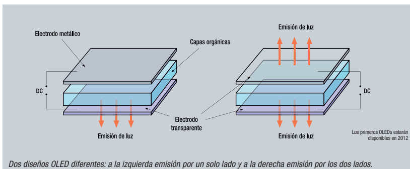
Dos diseños OLED diferentes: a la izquierda emisión por un solo lado y a la derecha emisión por los dos lados.
