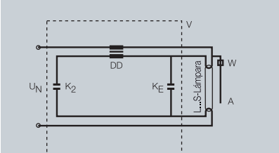
Fig. 5 Conexión semirresonante RD
