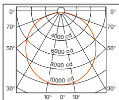
Diagrama polar
