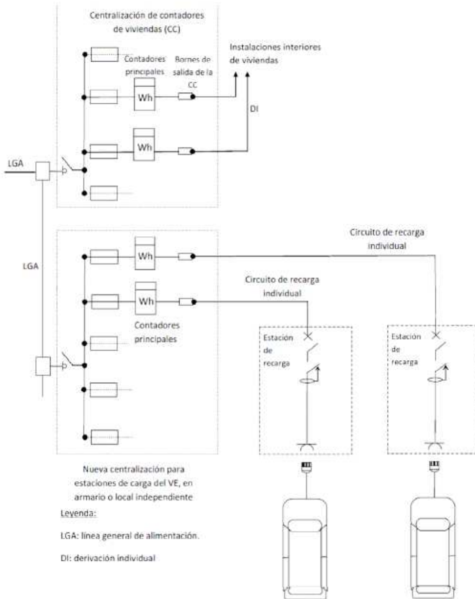
Figura 10. Esquema 3b: instalación individual con un contador principal para cada estación de recarga (con una nueva centralización de contadores).
